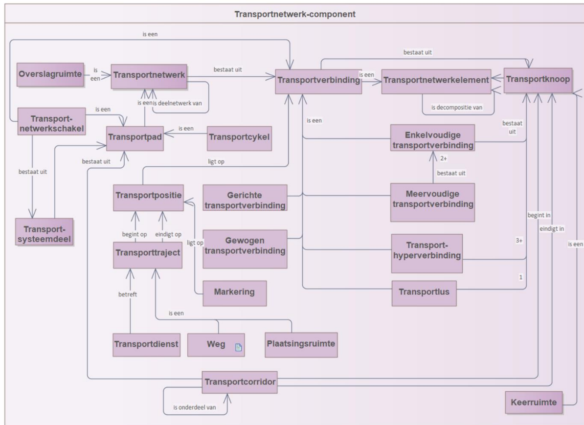
Figuur 7 Transportnetwerkinformatiemodel
