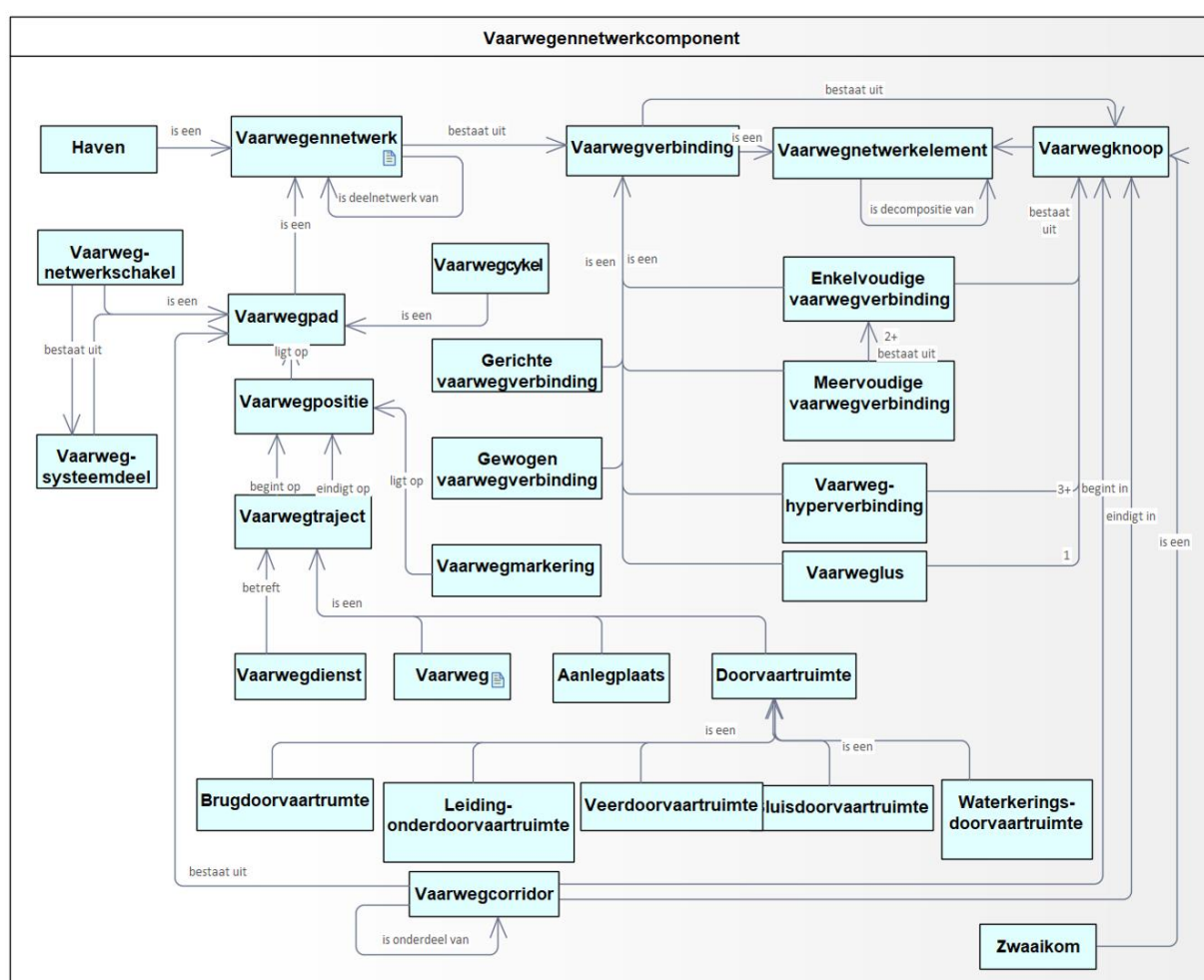
Figuur 8 Vaarwegennetwerkinformatiemodel
